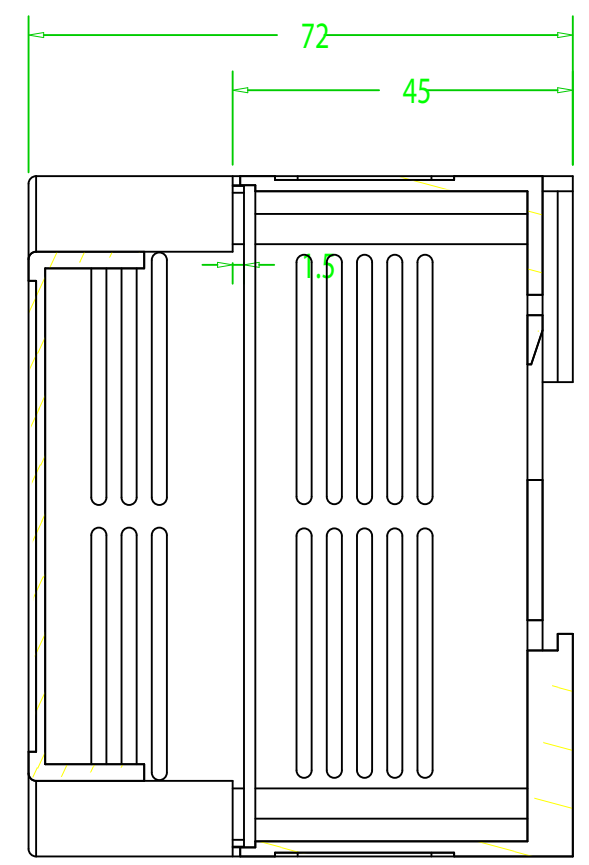
剖面 B-B
